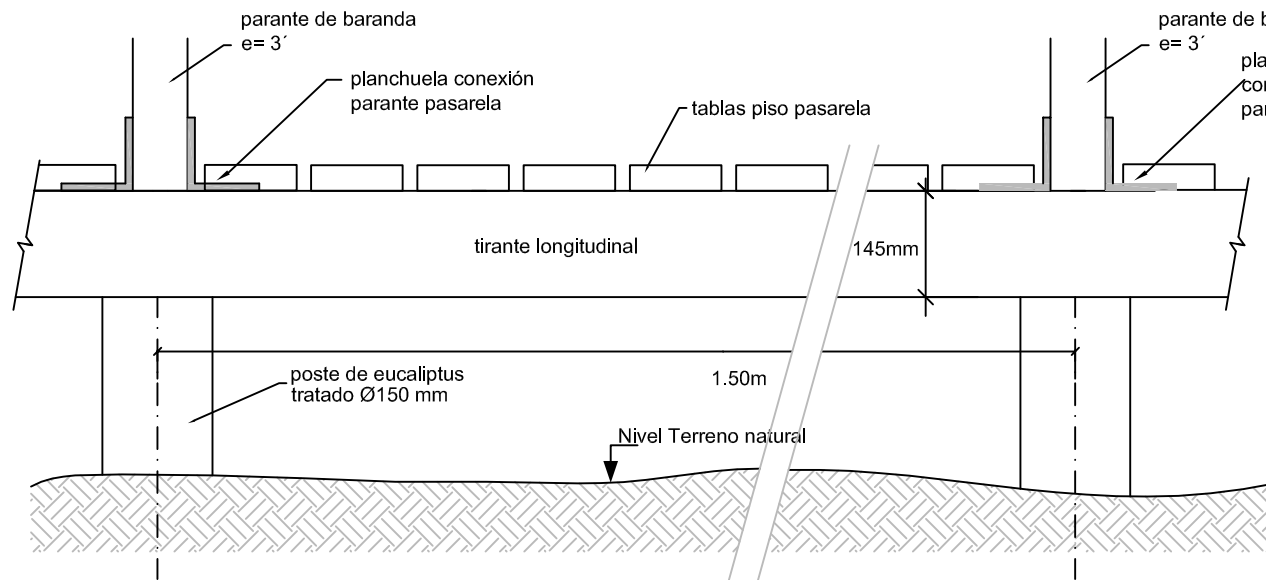
CORTE LONGITUDINAL
